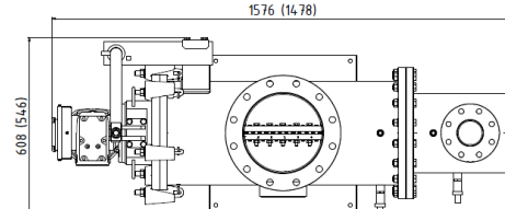
Dimensions in brackets without quick-change Abmessungen in Klammern ohne Schnellverschluss
